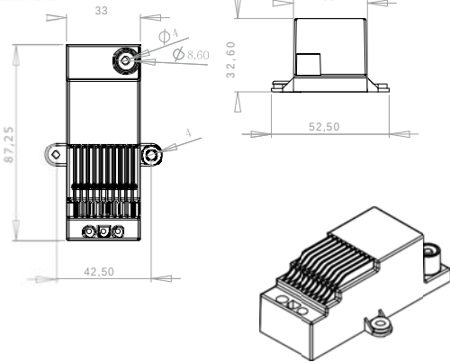
Technical drawing | Disegno tecnico [mm]
